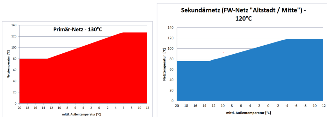
Abbildung 31: Netzvorlaufemperaturen im Heidelberger 130°C-Primärnetz links und im 120°C Sekundärnetz (rechts) nach TAB der SWHD 45
