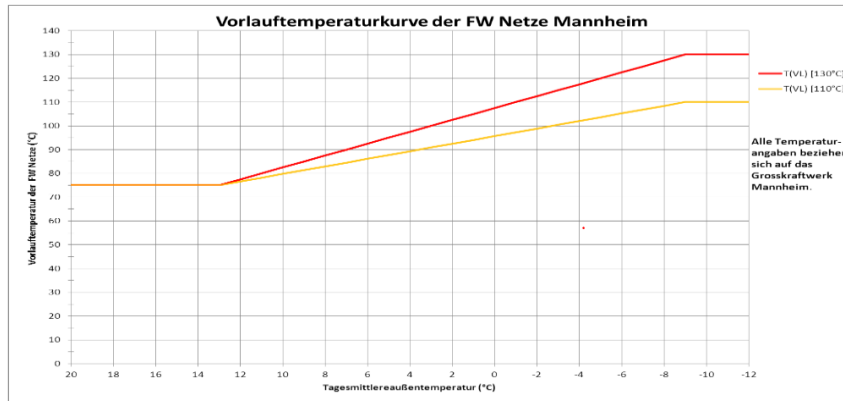
Abbildung 30: Netz-Vorlaufemperatur in den Mannheimer Wärmenetzen Abhängigkeit der Außentemperatur gemäß TAB der MVV 44 ()
