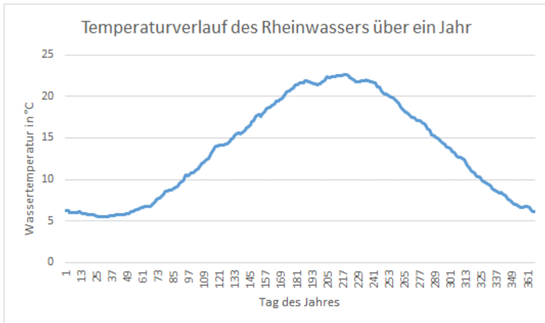
Abbildung 16: langjähriger Mittelwert der Wassertemperaturen des Rheins an der Messstelle Karlsruhe 16
