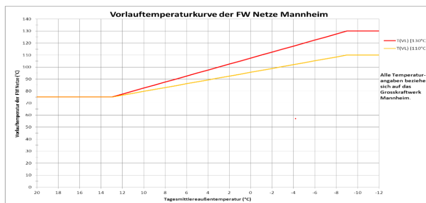
Abbildung 30: Netz-Vorlauftemperatur in den Mannheimer Wärmenetzen Abhängigkeit der Außentemperatur gemäß TAB der MVV 44 ()
