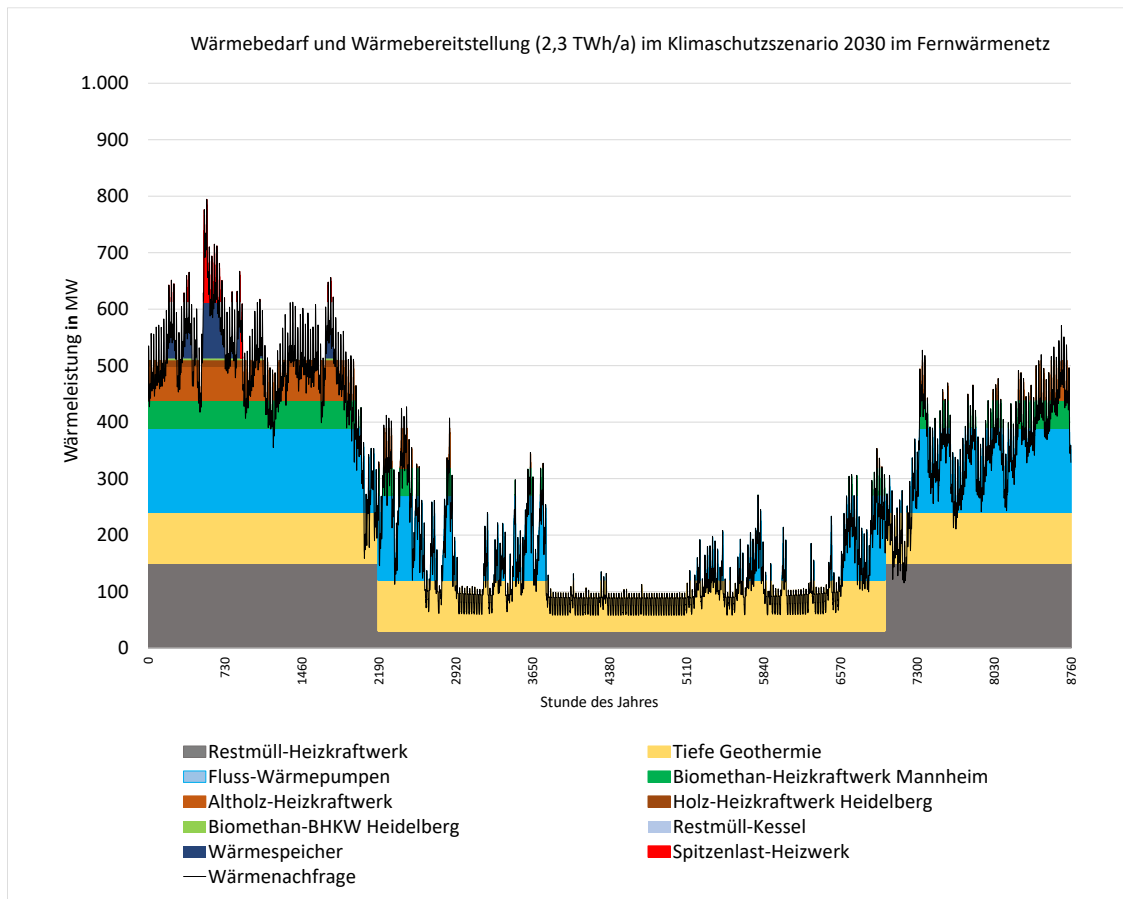
Abbildung 2: Wärmelastdeckung im Klimaschutzscenario 2030
