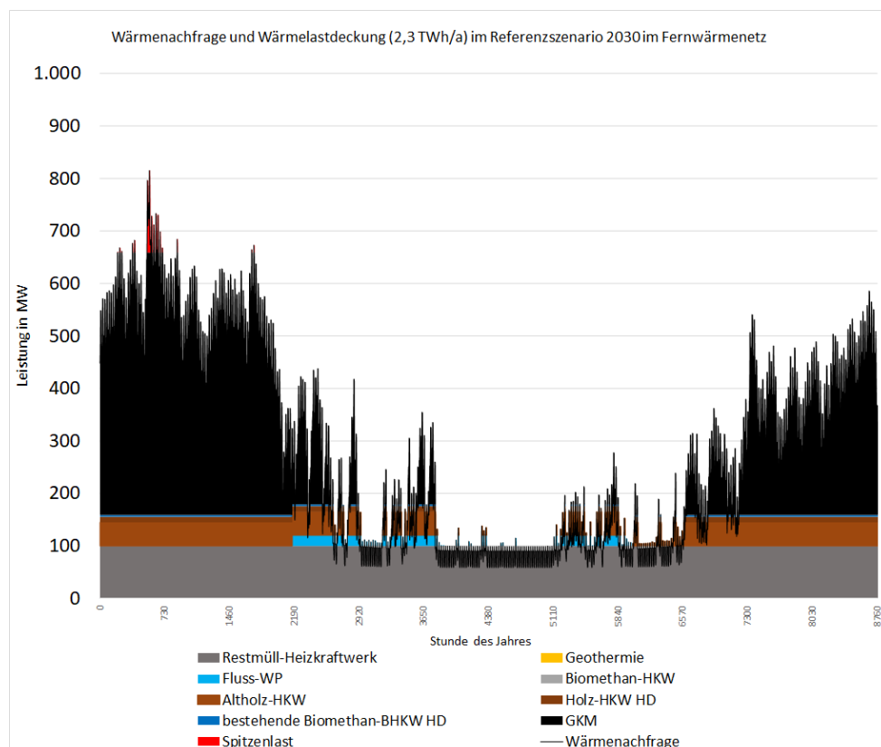
Abbildung 3: Wärmelastdeckung im Referenzscenario 2030
