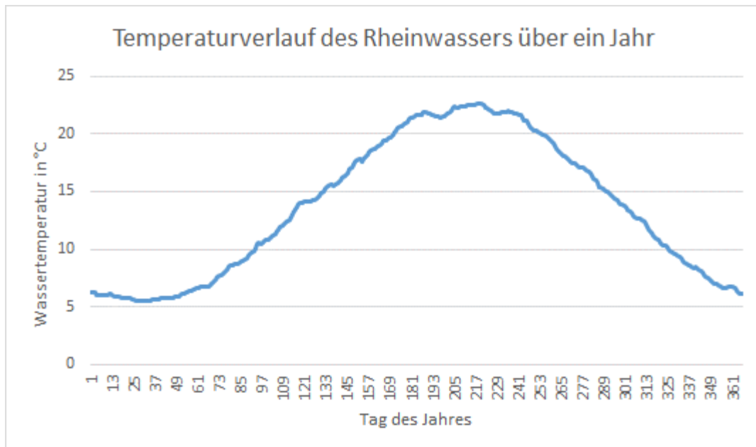
Abbildung 16: langjähriger Mittelwert der Wassertemperaturen des Rheins an der Messstelle Karlsruhe 16
