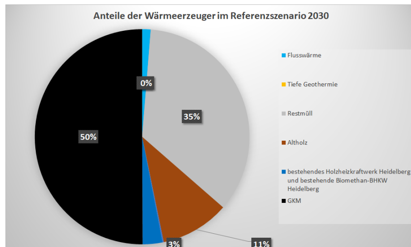
Abbildung 5: Anteile der Wärmeerzeuger an der Bereitstellung der Fernwärmenachfrage im Referenzscenario 2030
