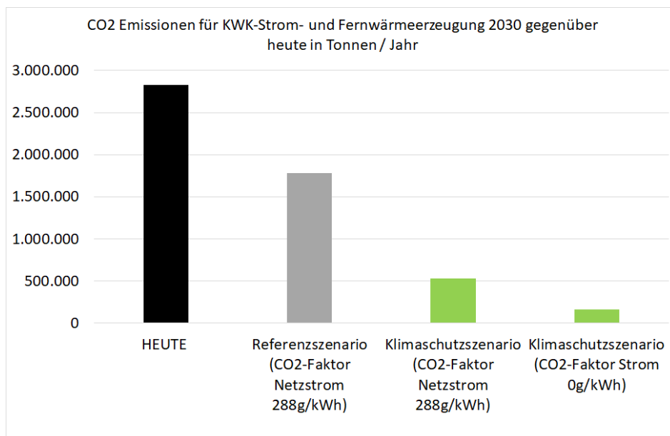
Abbildung 7: CO 2 -Emissionen für die Wärme- und (vermeidene) KWK-Stromerzeugung des GKM
