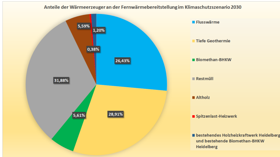
Abbildung 4: Anteile der Wärmeerzeuger an der Fernwärmebereitstellung im Jahr 2030 im Klimaschutzscenario
