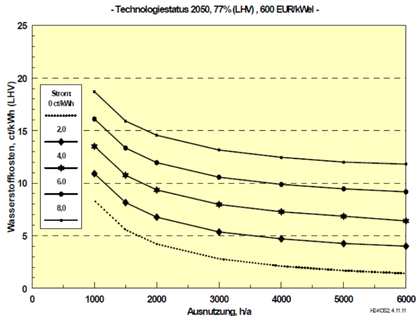
Abbildung 26: Gestehungskosten von Wasserstoff (am Elektrolyseur) bei verschiedenen Auslastungen der Anlage (y Achse) und Kosten für den Strom zur Wasserstofferzeugung gemäß der Einschätzung der BMU-Studie „Langfristszenarien für den Ausbau erneuerbarer Energien in Deutschland“ 42 , Zinssatz 6%/a, Abschreibung 20 a, Wartung/Betrieb 2% Inv./a, 77% Wirkungsgrad
