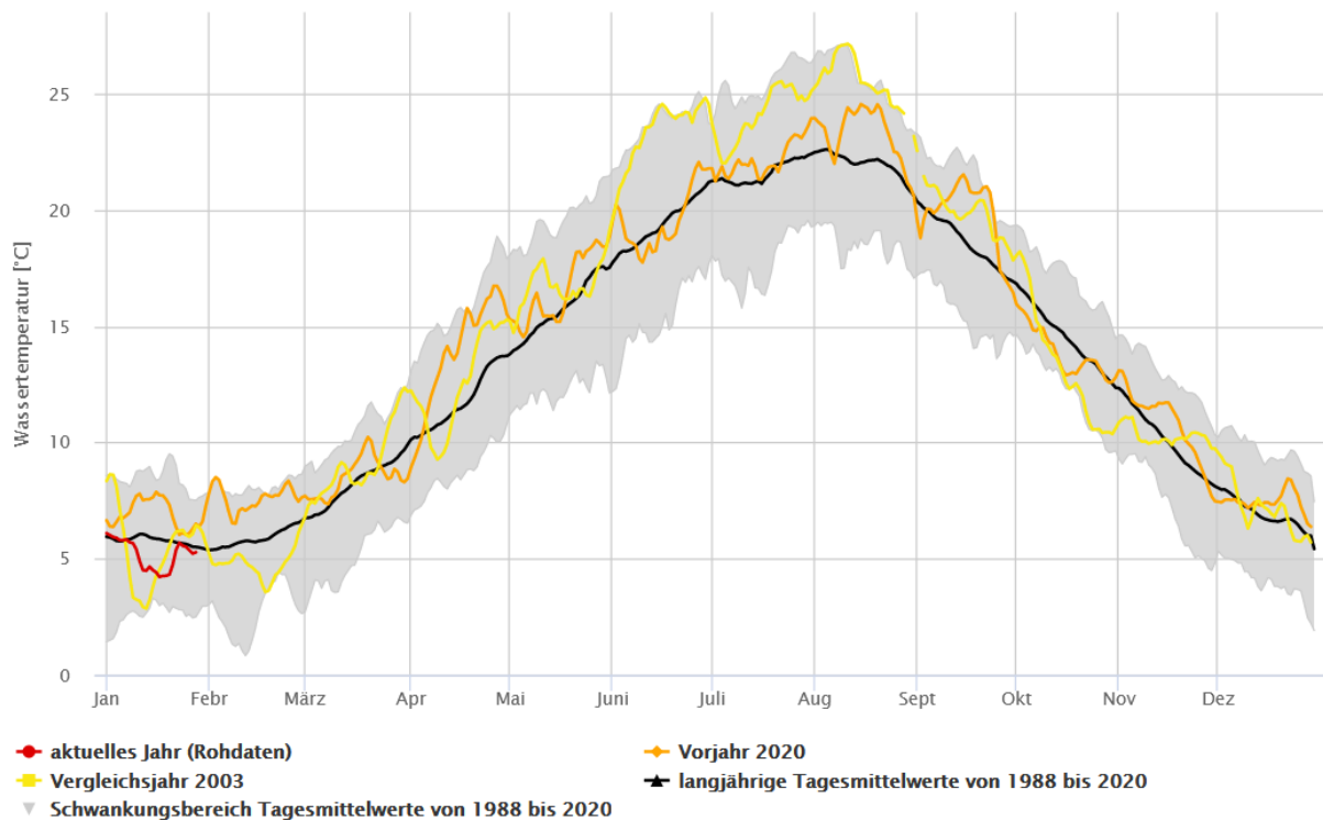
Abbildung 17: Mittlere Temperatur des Rheins am Messpegel Karlsruhe und ihre Schwankungsbreite zwischen 1988 und 2020
