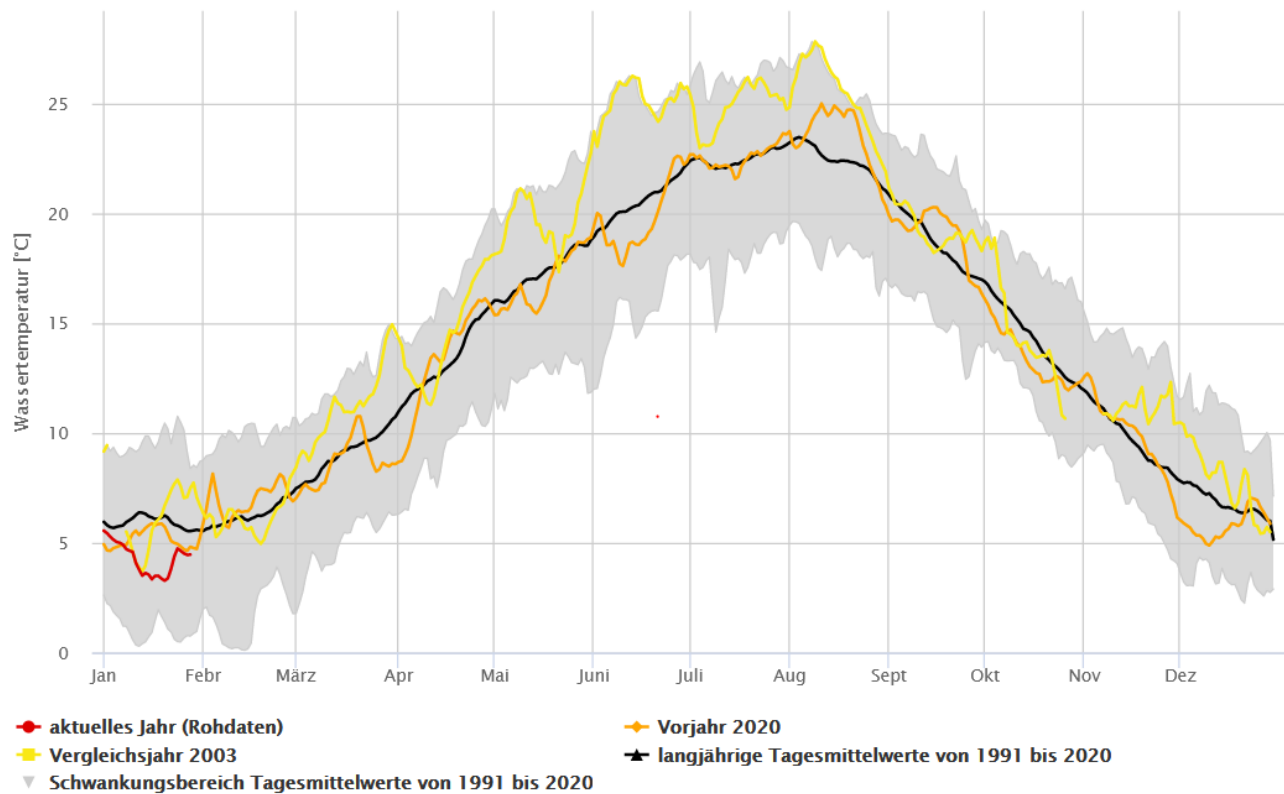
Abbildung 19: Temperaturverlauf des Neckarwassers und seine Schwankungsbreite am Messstandort Neckargemünd nach LUBW 18
