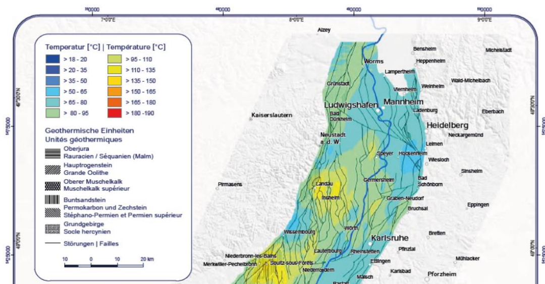
Abbildung 13: Temperaturen des Erdbodens und des Wassers in 1500 Meter unter der Erdoberfläche gemäß:
