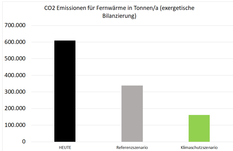
Abbildung 6: CO 2 -Emissionen der Wärmebereitstellung bei exergetischer Bilanzierung für KWK-Strom
