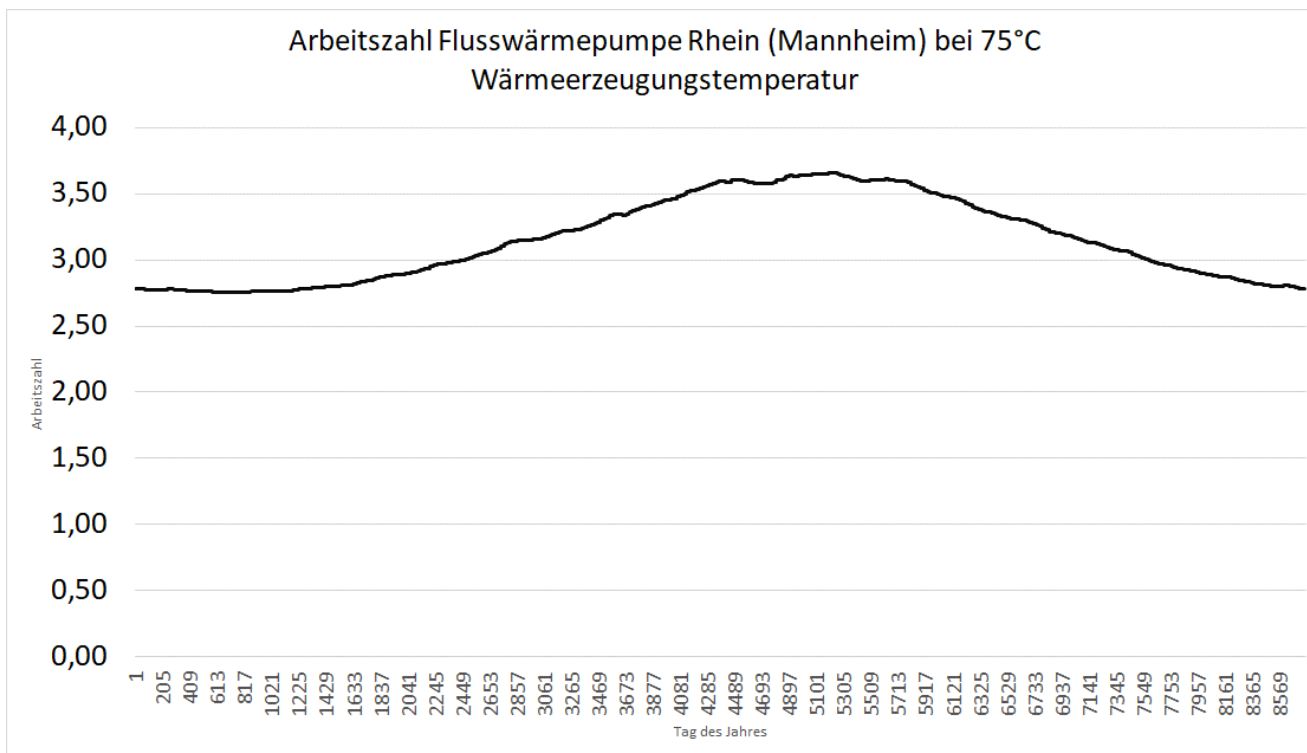
Abbildung 18: tägliche Arbeitszahl (= erzeugte Wärmemenge in kWh je eingesetzter kWh Strom) einer Rhein-Flusswärmepumpe bei einer Wärmeezeugungstemperatur von 75°C
